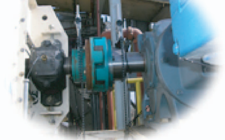
Alineacion FAS LP en transportador
